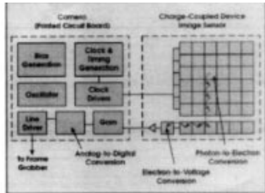
تالیه‌تی گواسته‌وه‌ی چارج له CCD
